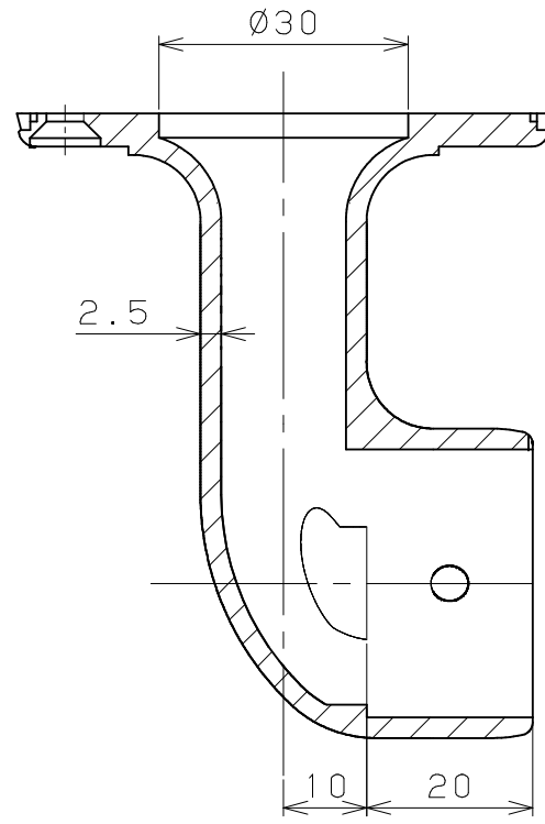
A-A断面図
